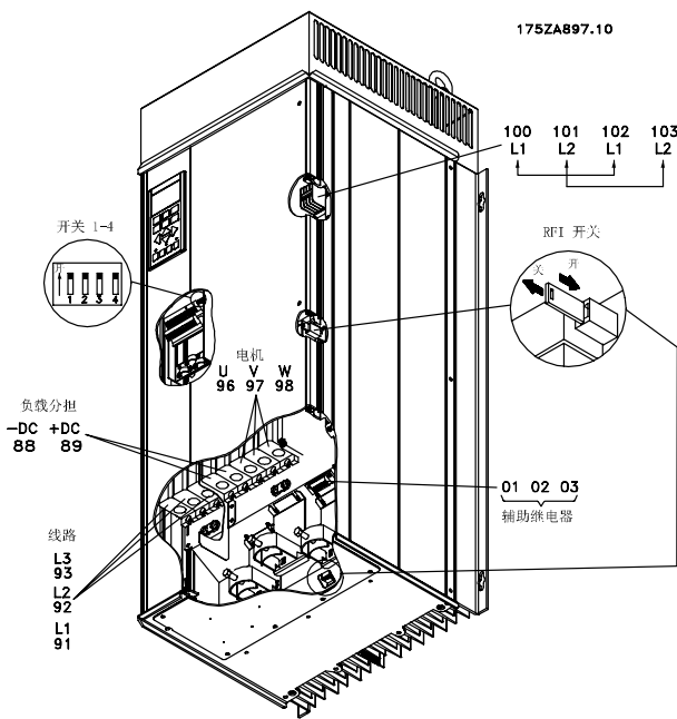
紧凑型 IP 54 VLT 6102-6122, 380-460 V
