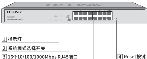
图1-4 TL-SG2016前面板示意图
