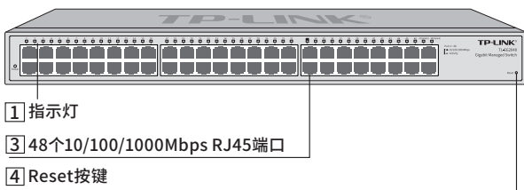
图1-1 TL-SG2048前面板示意图
