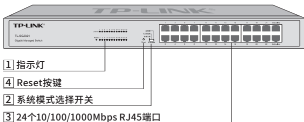
图1-2 TL-SG2024前面板示意图
