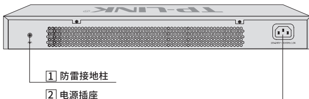
图1-7 TL-SG2048后面板示意图
