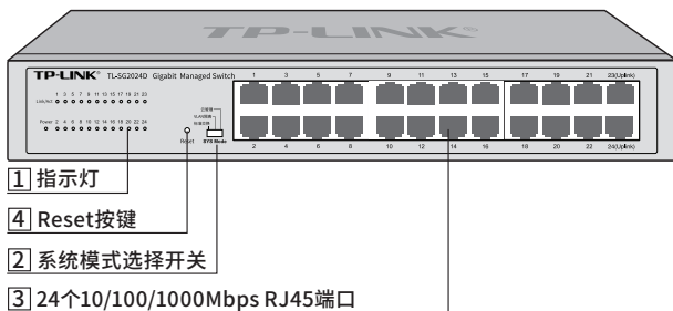
图1-3 TL-SG2024D前面板示意图
