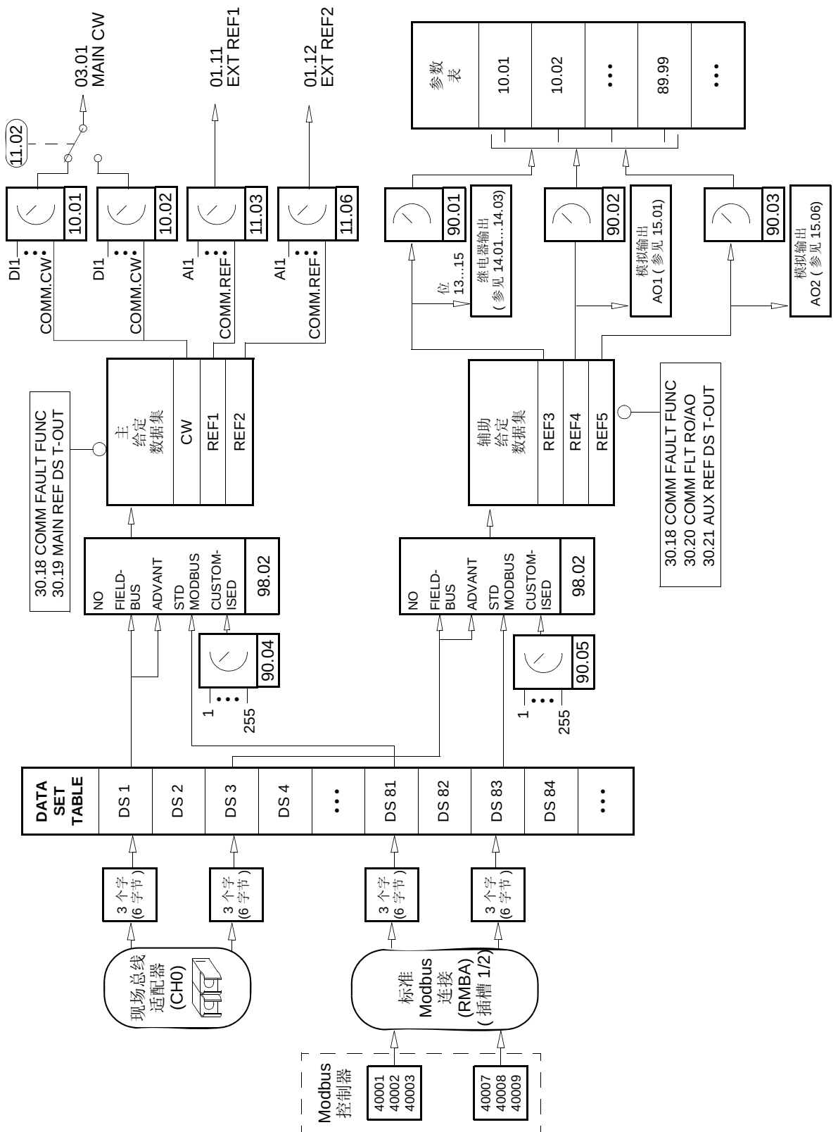
方框图：使用 Nxxx 型现场总线适配器时，来自现场总线的控制数据的输入
