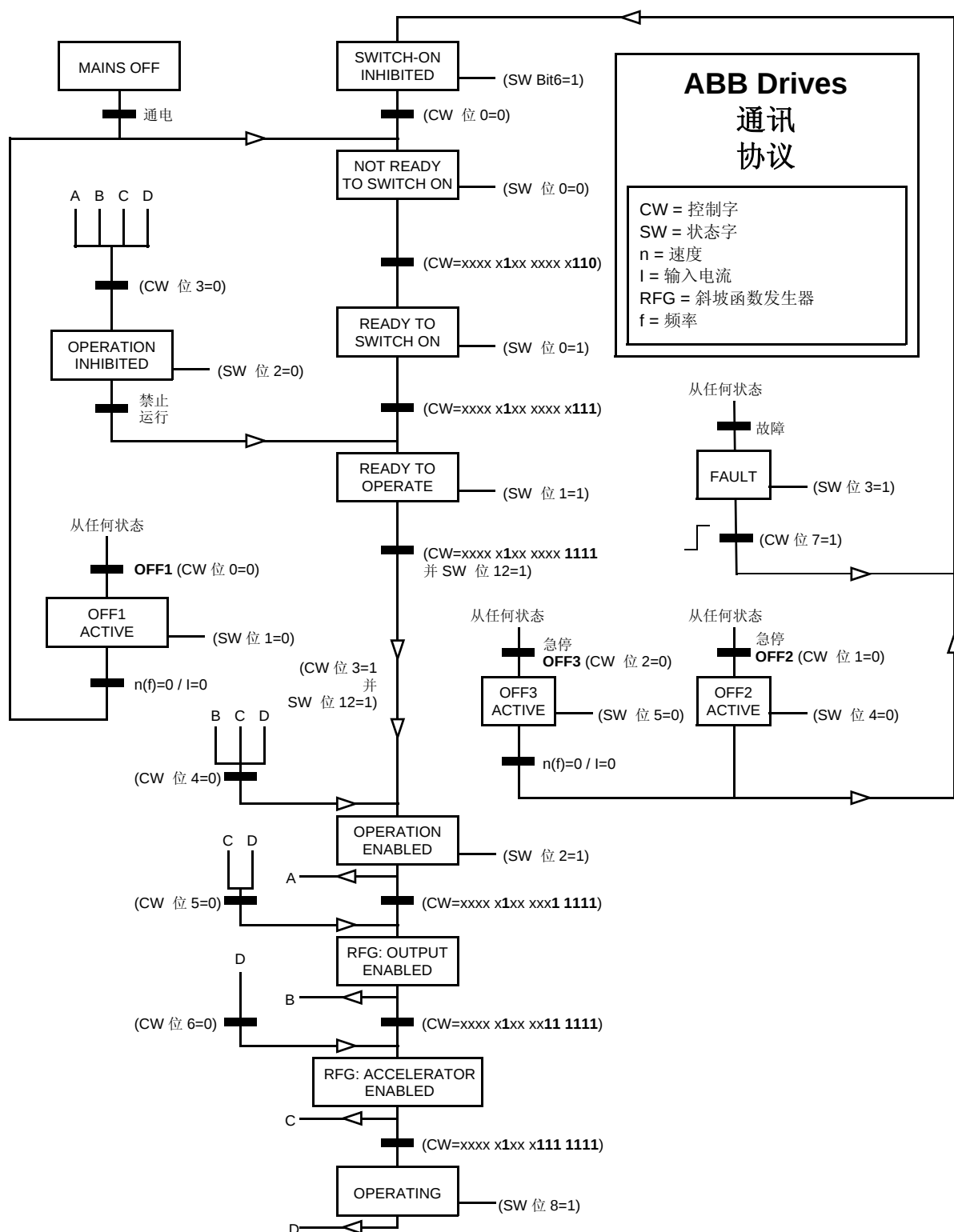
图1 ABB Drives 通讯协议的状态机器
