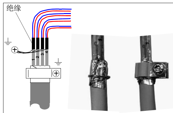
双屏蔽电缆
